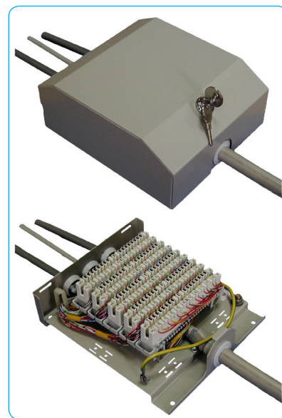
Коробка КР-50М
