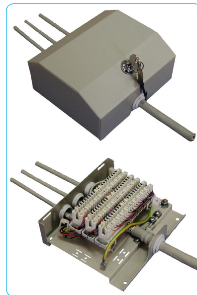
Коробка КР-30М
