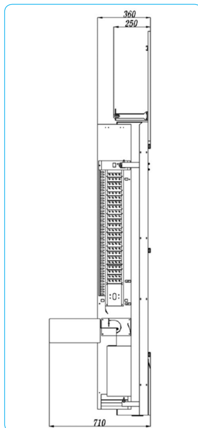
Стойка СОКР-2,2М в раскрытой позиции. Кассета развернута для монтажа
