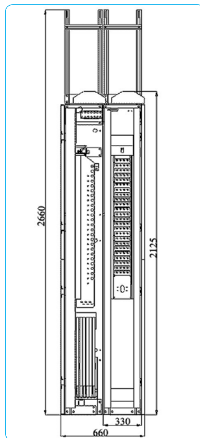
Две стойки СОКР-2,2М в ряду. Левая стойка в раскрытой позиции
